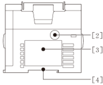
右侧面
